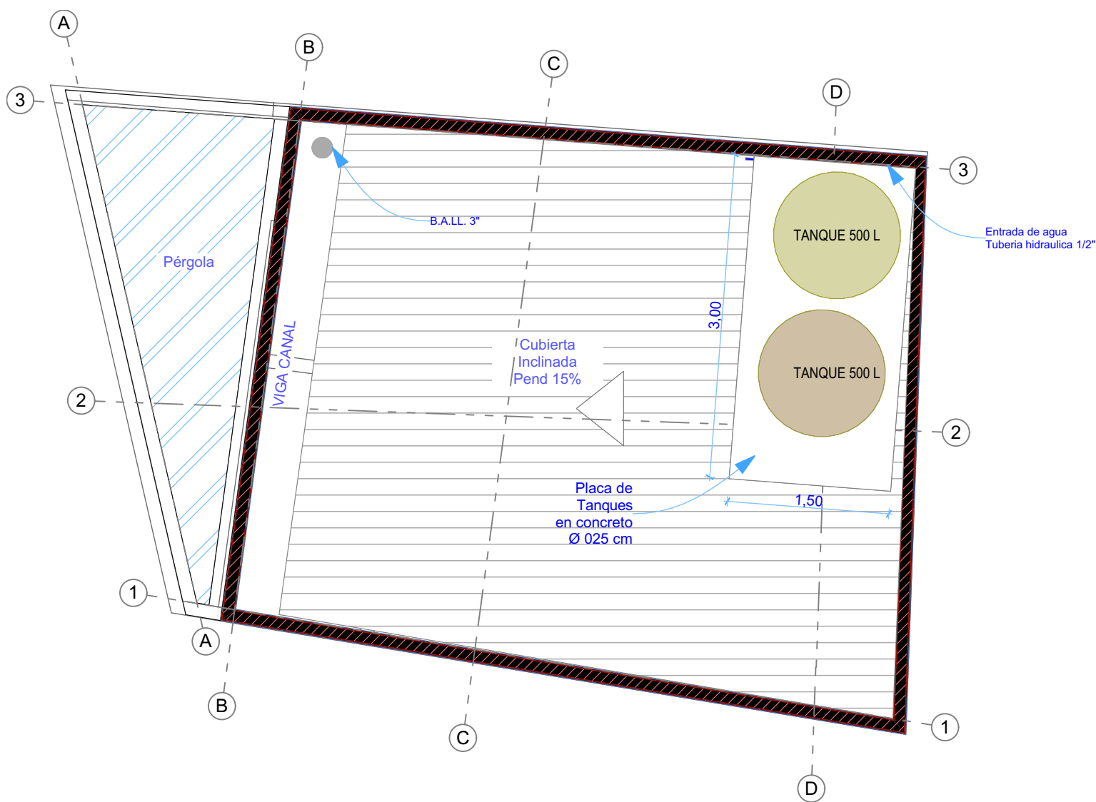
HIDROSANITARIO DE CUBIERTAS ESC 1:50
