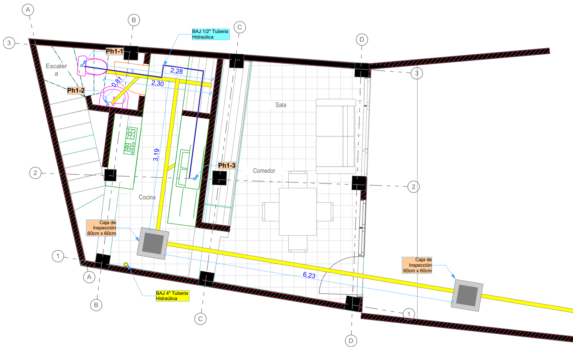
HIDROSANITARIO DE PRIMER PISO ESC 1:50
