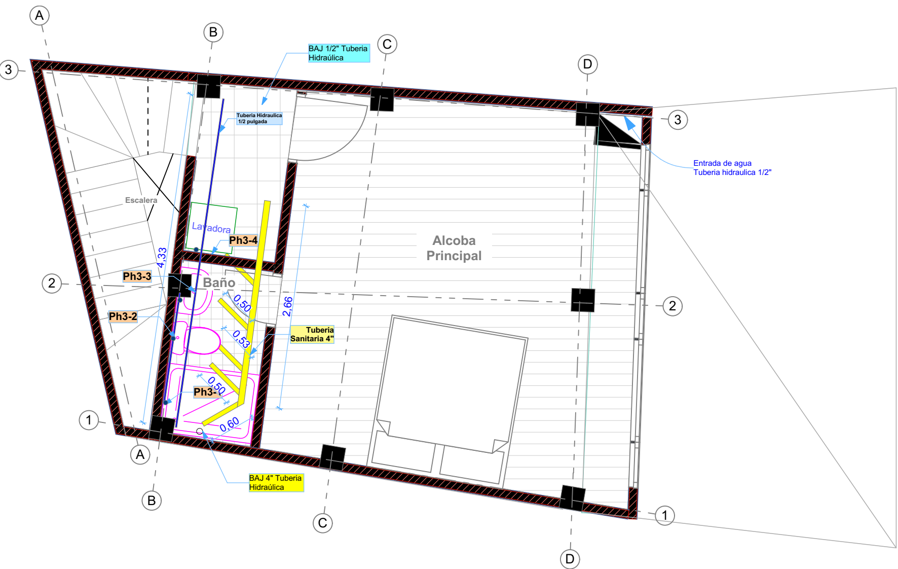
HIDROSANITARIO DE TERCER PISO ESC 1:50
