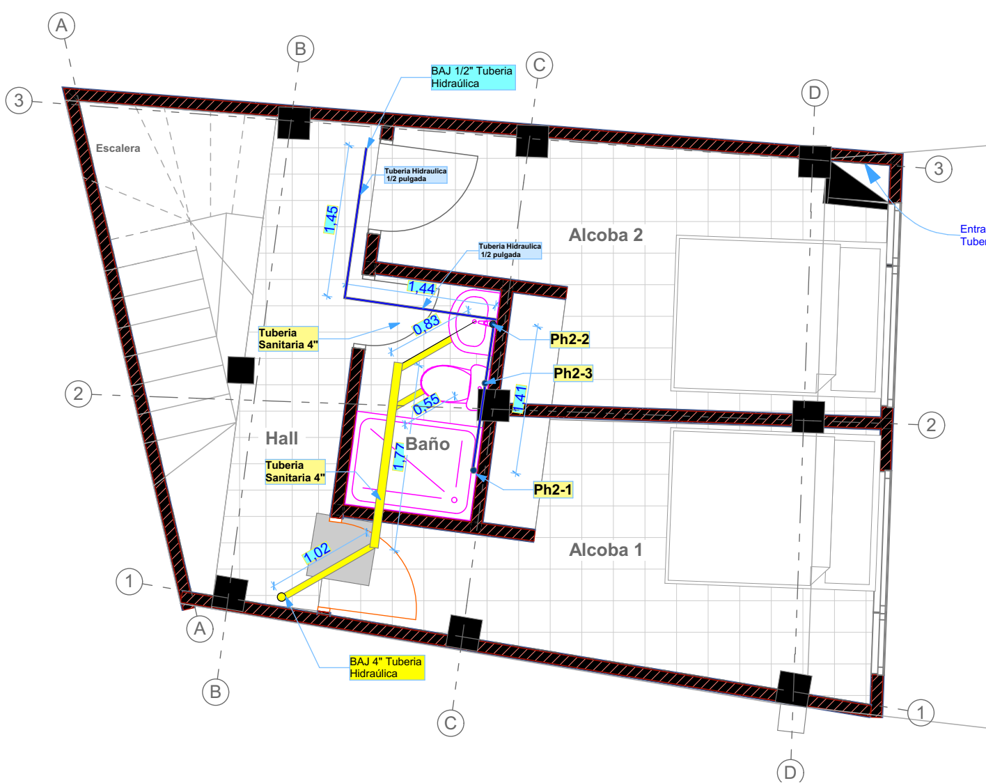
HIDROSANITARIO DE SEGUNDO PISO ESC 1:50
